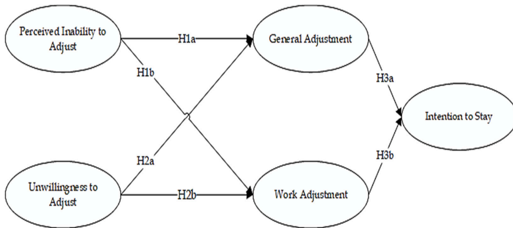
Gambar 1 Kerangka Pemikiran
